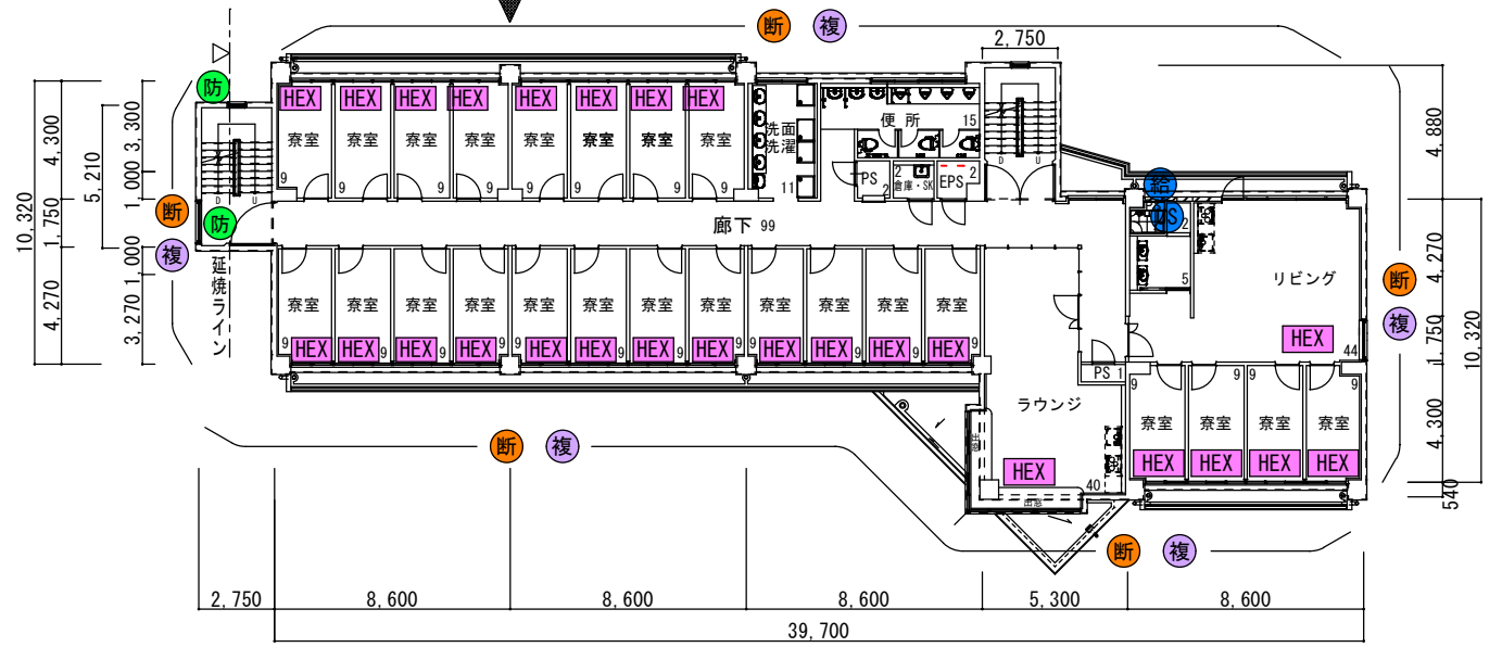
2～5階平面図 S=1:300 (改修前)
