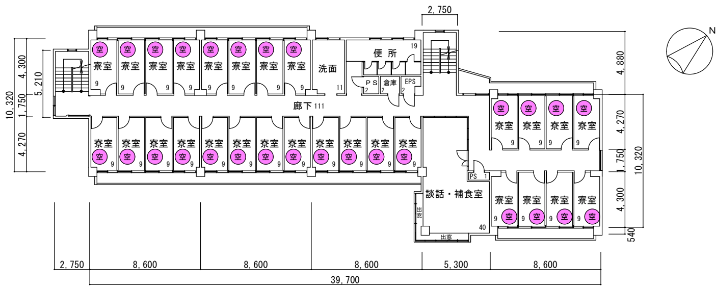
2～5階平面図 S=1:300 (改修前)
