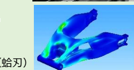
鈴鹿8耐参戦用モーターバイクの応力解析(スイングアーム)
