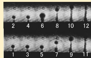
(a) Si 3 N 4 の衝撃破壊(T=1000℃, 10 6 コマ毎秒)
