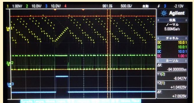
左の回路で観測された電荷平衡型+シングルスロープ型A/D変換の波形
