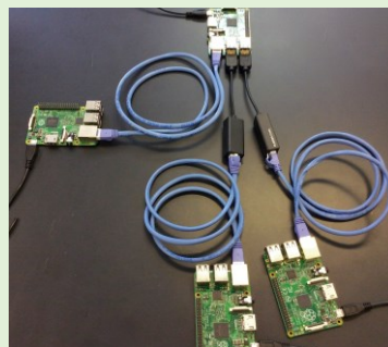
RaspberryPiを用いた通信実験デバイス
